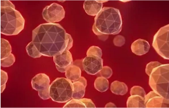
QUIONE: a quantum simulator
