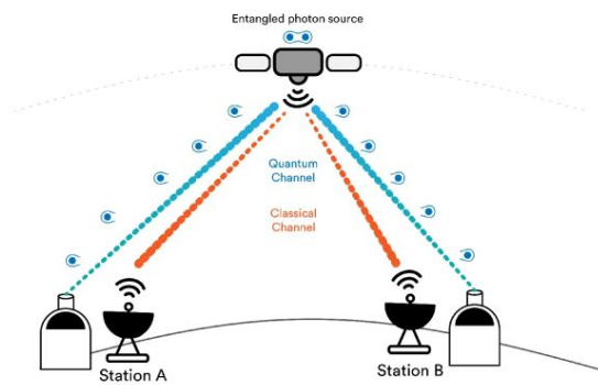
Transmisión de QKD en el espacio libre utilizando una fuente de fotones entrelazados
