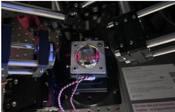
Guía de ondas utilizada en el estudio. Credito: ICFO.
