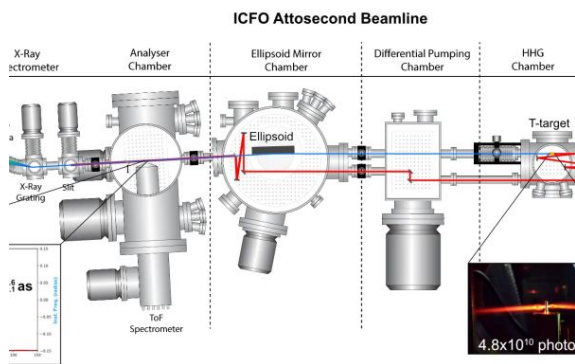
Esquema del diseño experimental de ICFO para generar, acondicionar y analizar pulsos de rayos X de attosegundos. El diagrama sigue la propagación del haz laser infrarrojo (rojo) y del haz de rayos X blandos (azul).
