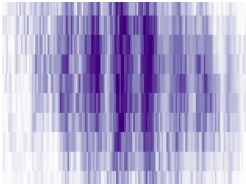
Imagen experimental in situ del perfil de densidad de la nube de átomos de potasio, medida mediante
