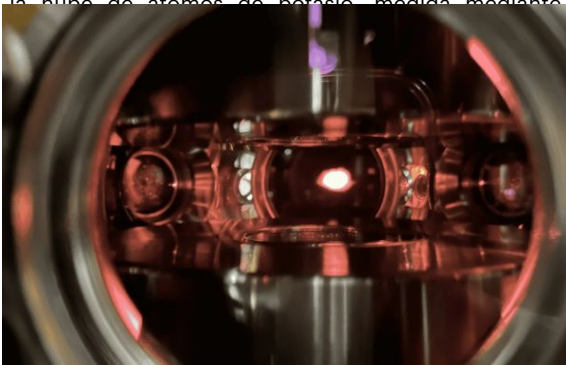
Átomos de potasio en la trampa magneto-óptica, una etapa intermedia antes de la formación de un condensado de Bose-Einstein. ©ICFO.
